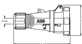
Ölçüler (mm)
