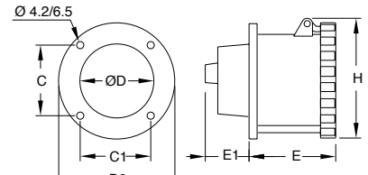
Ölçüler (mm)
